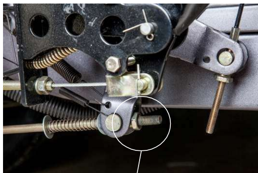
Регулировочная гайка заднего тормоза
