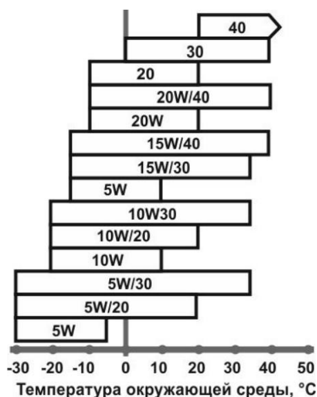
Рисунок 5.2. Классификация масел
