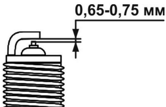
Рисунок 5.6. Свеча зажигания, регулировка зазора
