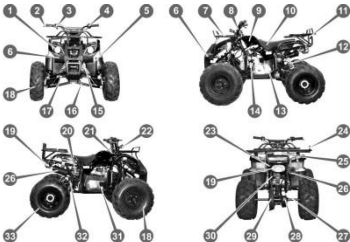
Рисунок 3.1. Расположение узлов и агрегатов
