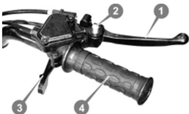
Рисунок 3.5. Блок переключателей правый
